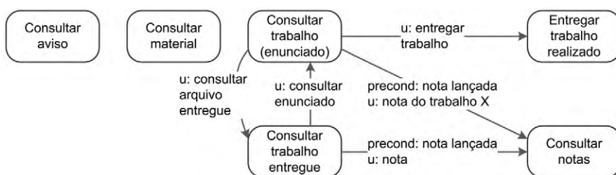
Figura 7.7 Diagrama (parcial) de interação do aluno com falas de transição de usuário.
