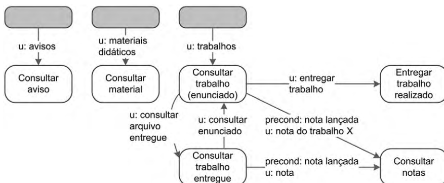
Figura 7.8 Diagrama (parcial) de interação do aluno, incluindo os acessos ubíquos.
