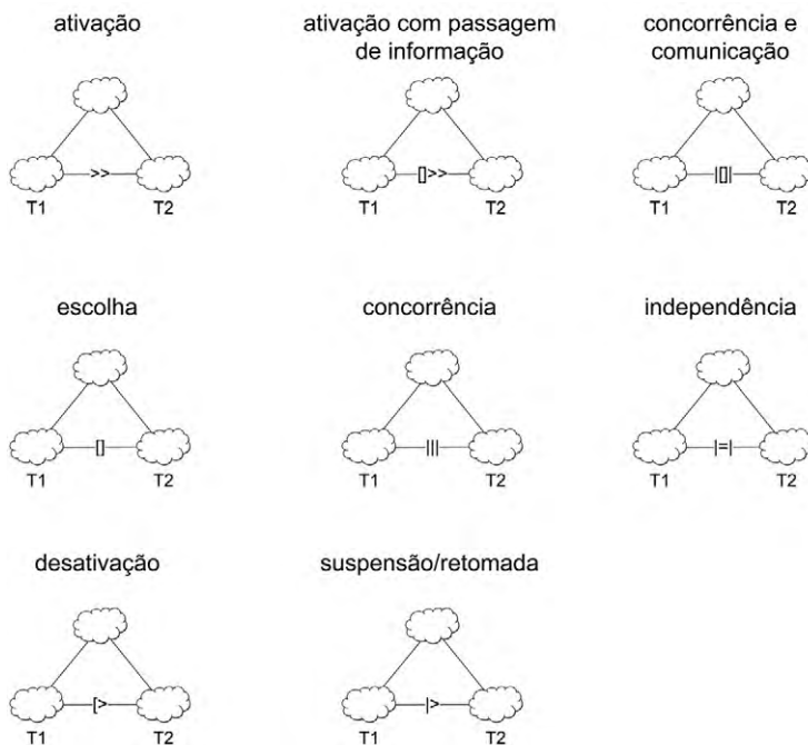
Figura 6.5 Relações entre tarefas no CTT.
