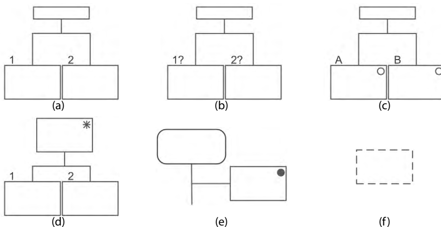
Figura 7.5 Representação de estrutura de tarefa (a) sequencial, (b) independente de ordem, (c) alternativa, (d) iterativa, (e) ubíqua e (f) opcional.
