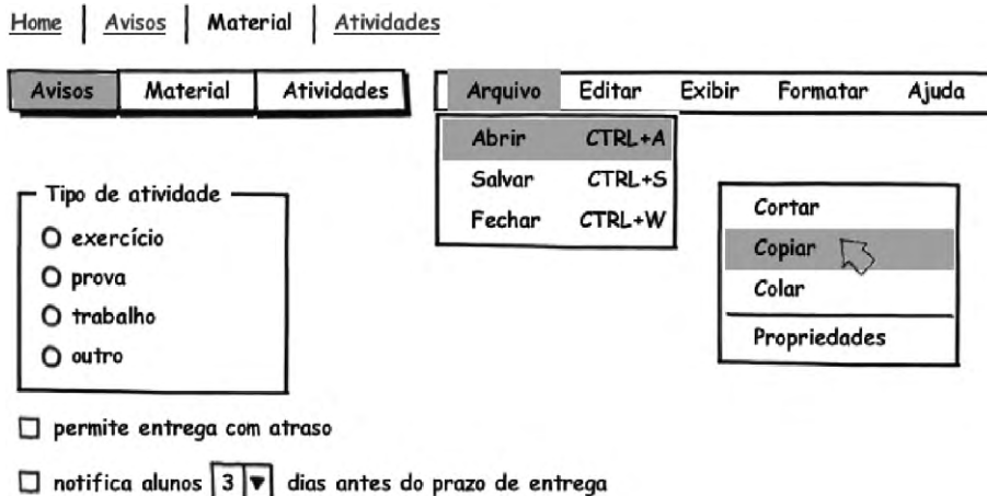
Figura 7.19 Exemplos de diferentes formas de menu.
