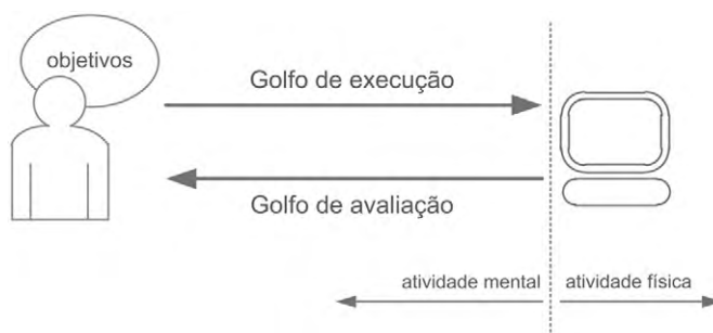
Figura 3.15 Golfos de execução e de avaliação que o usuário precisa atravessar ao interagir com um sistema físico.
