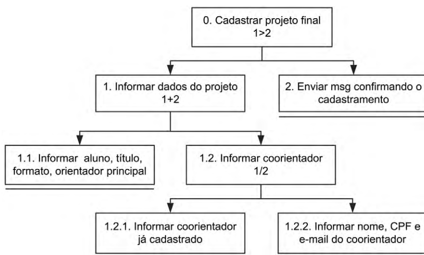
Figura 6.2 Diagrama HTA, para o objetivo de cadastrar um projeto final em um sistema acadêmico.
