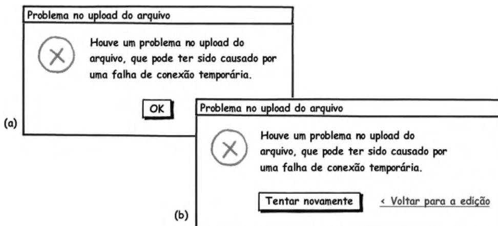
Figura 8.9 Exemplo de mensagens de erro (a) sem e (b) com oportunidade de recuperação e retomada de um caminho de interação produtivo.
