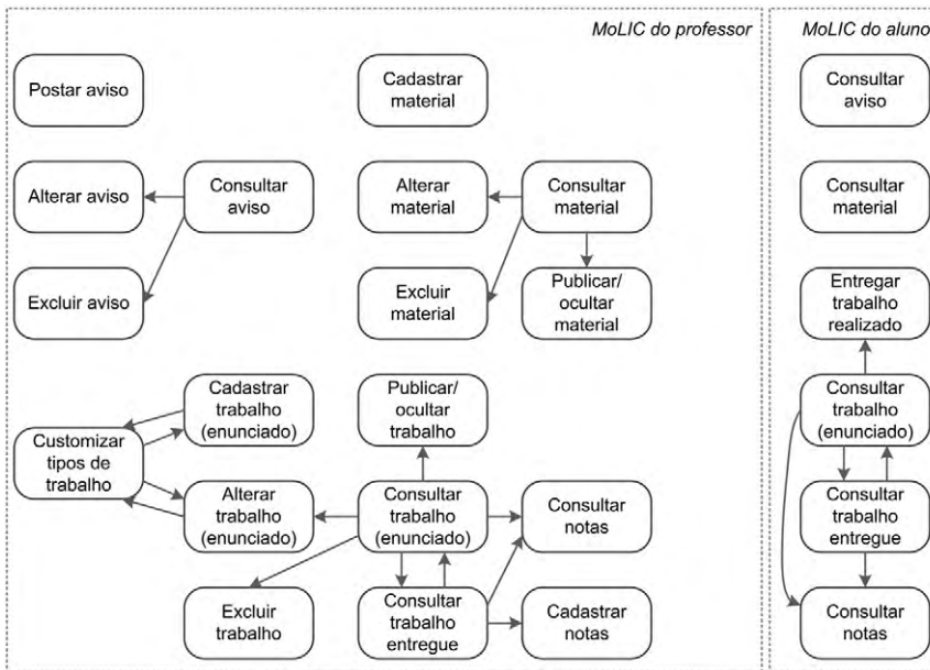
Figura 7.6 Diagramas parciais de interação do professor e do aluno, cujos tópicos foram extraídos do mapa de objetivos.
