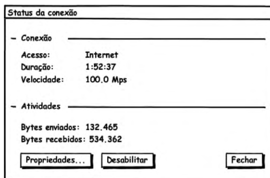
Figura 8.8 Posicionamento de um botão de uso frequente (Propriedades) próximo a um botão de uso infrequente e consequências graves (Desabilitar).
