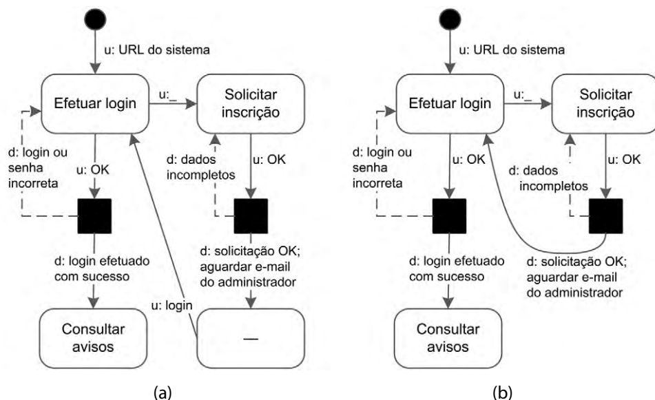
Figura 7.12 Resposta do preposto do designer sobre um processamento, a) sem mudança de tópico; b) com mudança de tópico.
