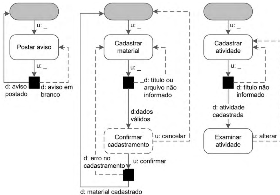
Figura 7.14 Diferentes tipos de conversa para o cadastramento de aviso, material didático e atividade.
