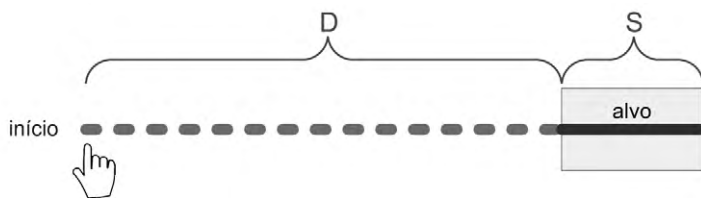
Figura 3.1 Ilustração da lei de Fitts.
