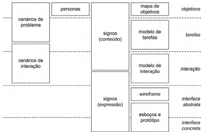
Figura 7.1 Representações utilizadas para explorar diferentes aspectos de IHC.
