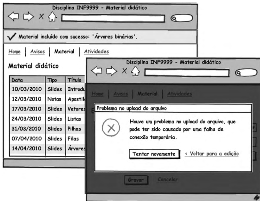
Figura 8.7 Feedback sutil e destacado.
