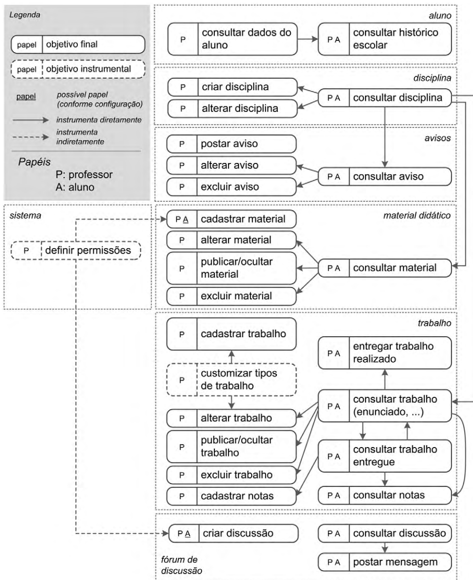
Figura 7.2 Mapa de objetivos dos usuários.
