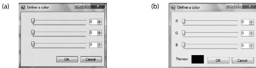
Figura 3.13 Diálogos para escolha de cores ilustrando problemas de mapeamento, controle e avaliação.
