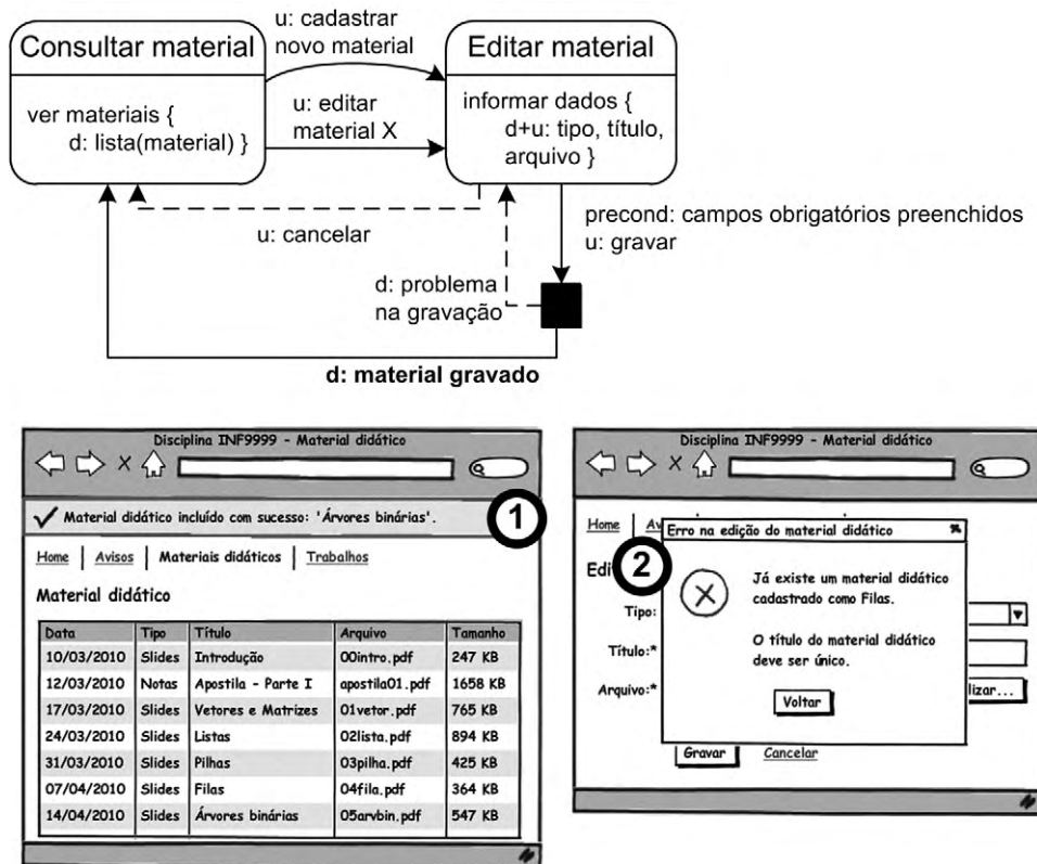
Figura 7.30 Falas de transição do preposto do designer mapeadas para elementos de interface.
