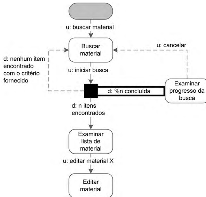
Figura 7.11 Processo do sistema e comunicação consecutiva e síncrona.
