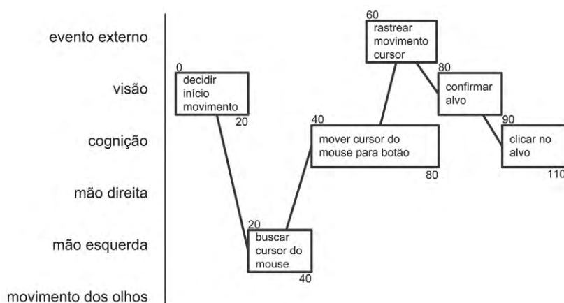
Figura 6.3 Exemplo de modelo CPM-GOMS.
