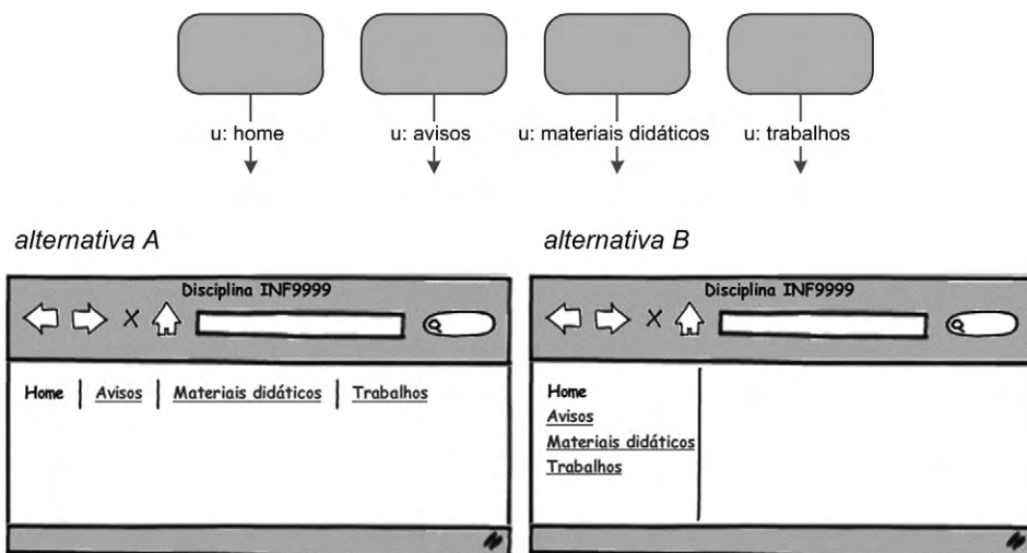
Figura 7.26 Acessos ubíquos mapeados para uma barra de navegação, considerando duas alternativas: (a) horizontal e (b) vertical.
