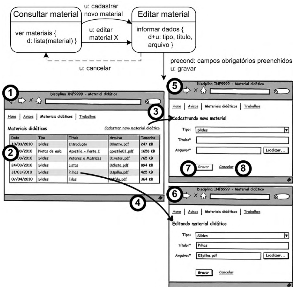
Figura 7.29 Diálogos e signos mapeados em elementos de interface.
