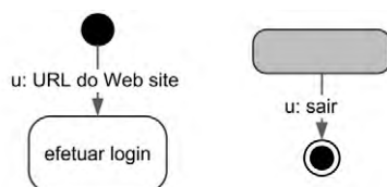
Figura 7.9 Diagrama (parcial) de interação do aluno, incluindo os pontos de abertura e encerramento da conversa usuário–preposto.
