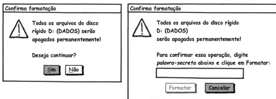
Figura 8.4 Diálogos de confirmação para uma operação que não pode ser desfeita. Qual é a mais segura?
