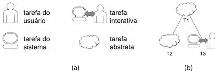
Figura 6.4 Representações (a) dos tipos de tarefas e (b) da sua hierarquia no CTT.
