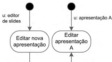
Figura 7.10 Pontos de abertura da conversa global usuário–preposto em um editor de apresentações (diagrama parcial).
