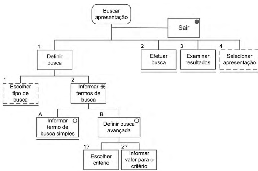
Figura 7.4 Modelo hierárquico de tarefas adaptado.
